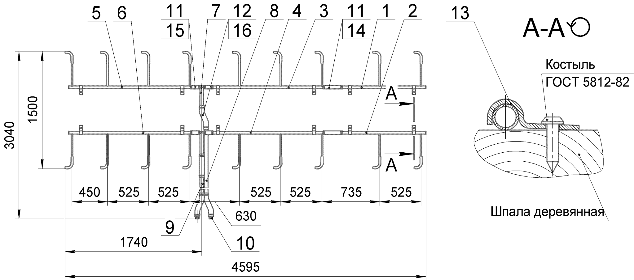
Рисунок 1. Арматура пневматической очистки стрелок АС-50Д
